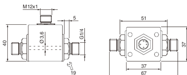
▶外形寸法図(単位:mm)
