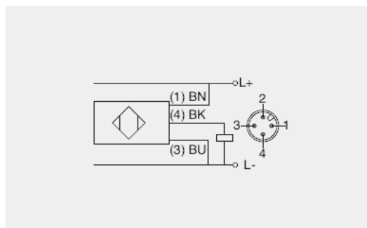
▶結線図
