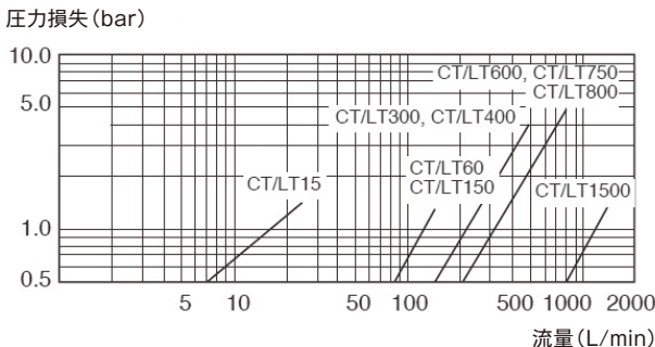
標準21cSt時の圧力損失表
